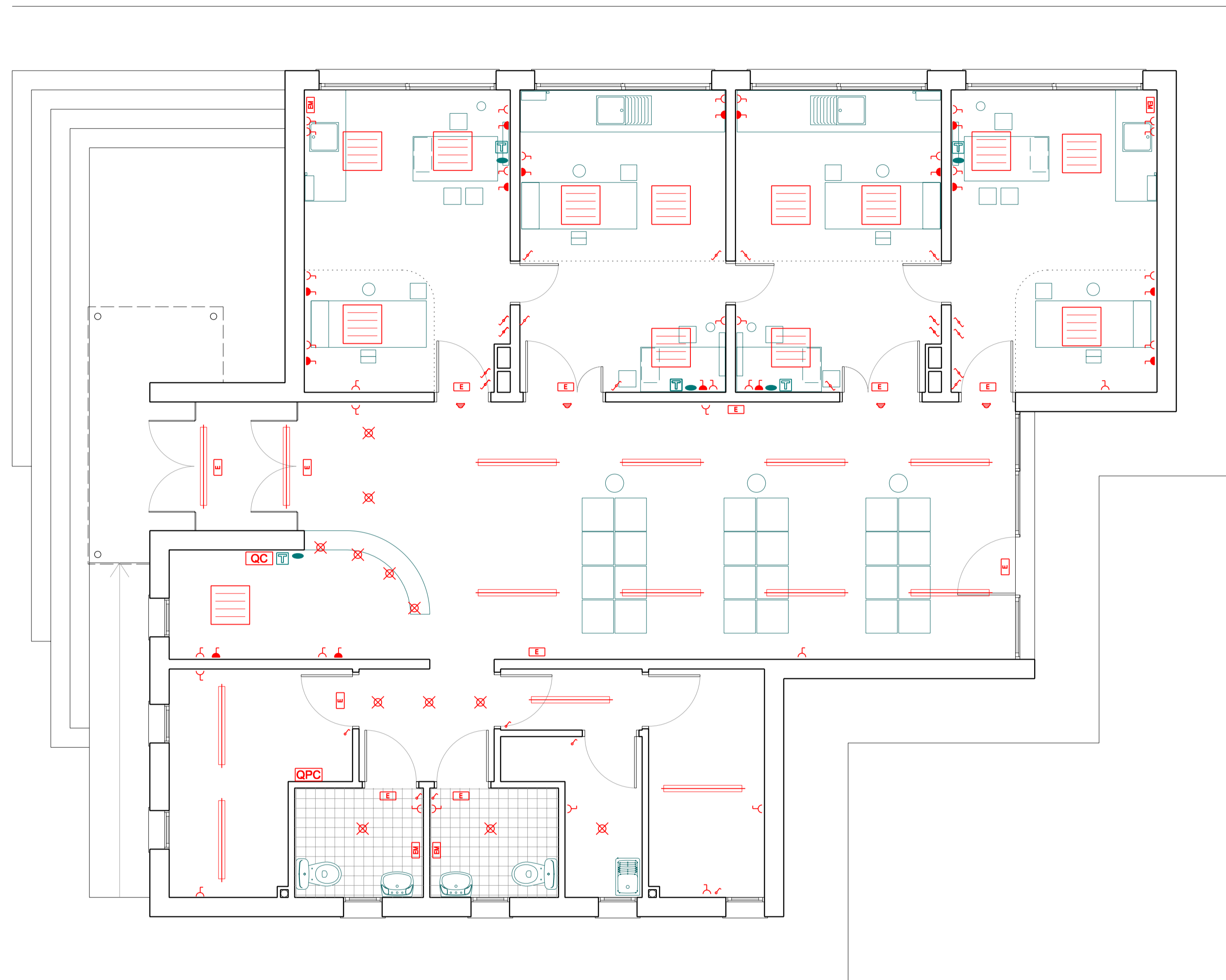
PLANTA D'INSTAL·LACIONS
