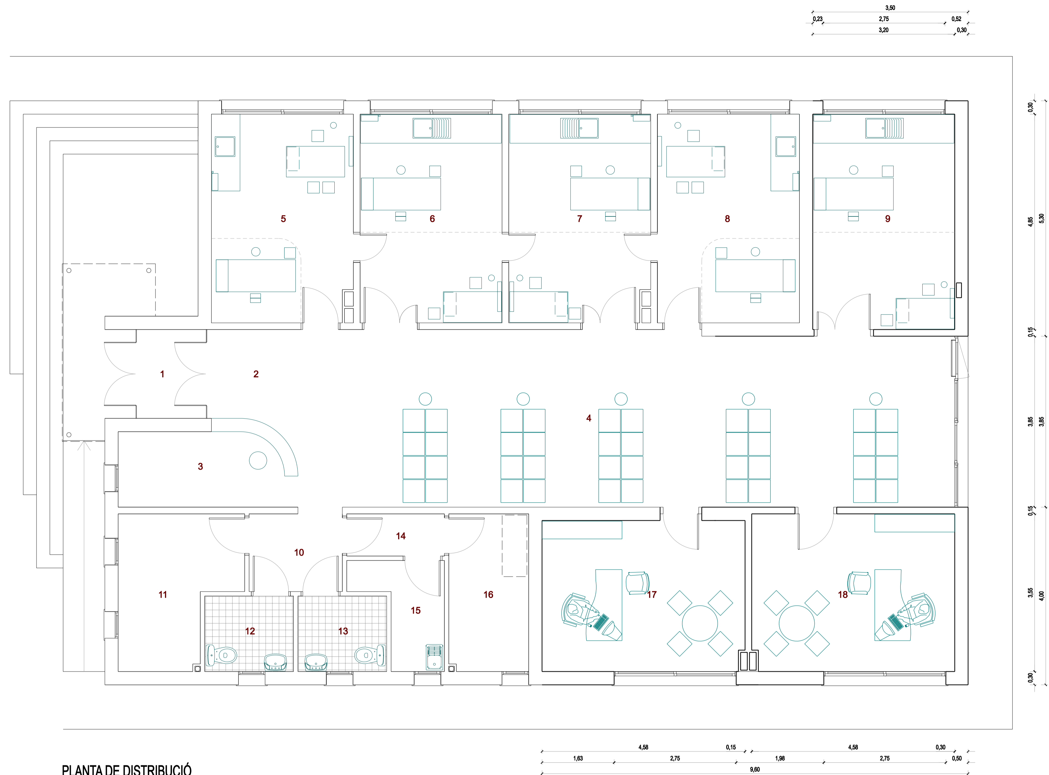
PLANTA DE DISTRIBUCIÓ
