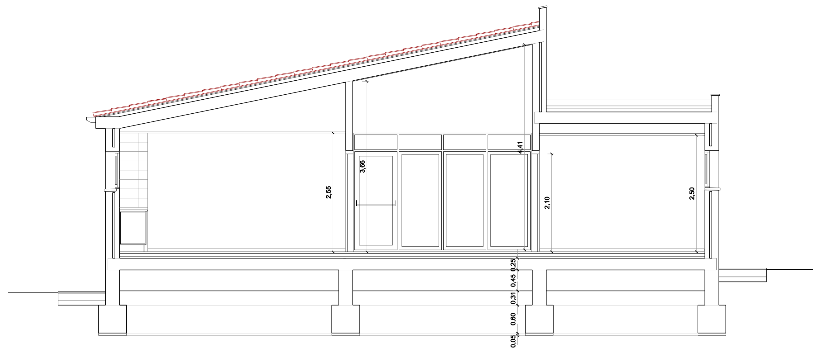
SECCIÓ AA'
